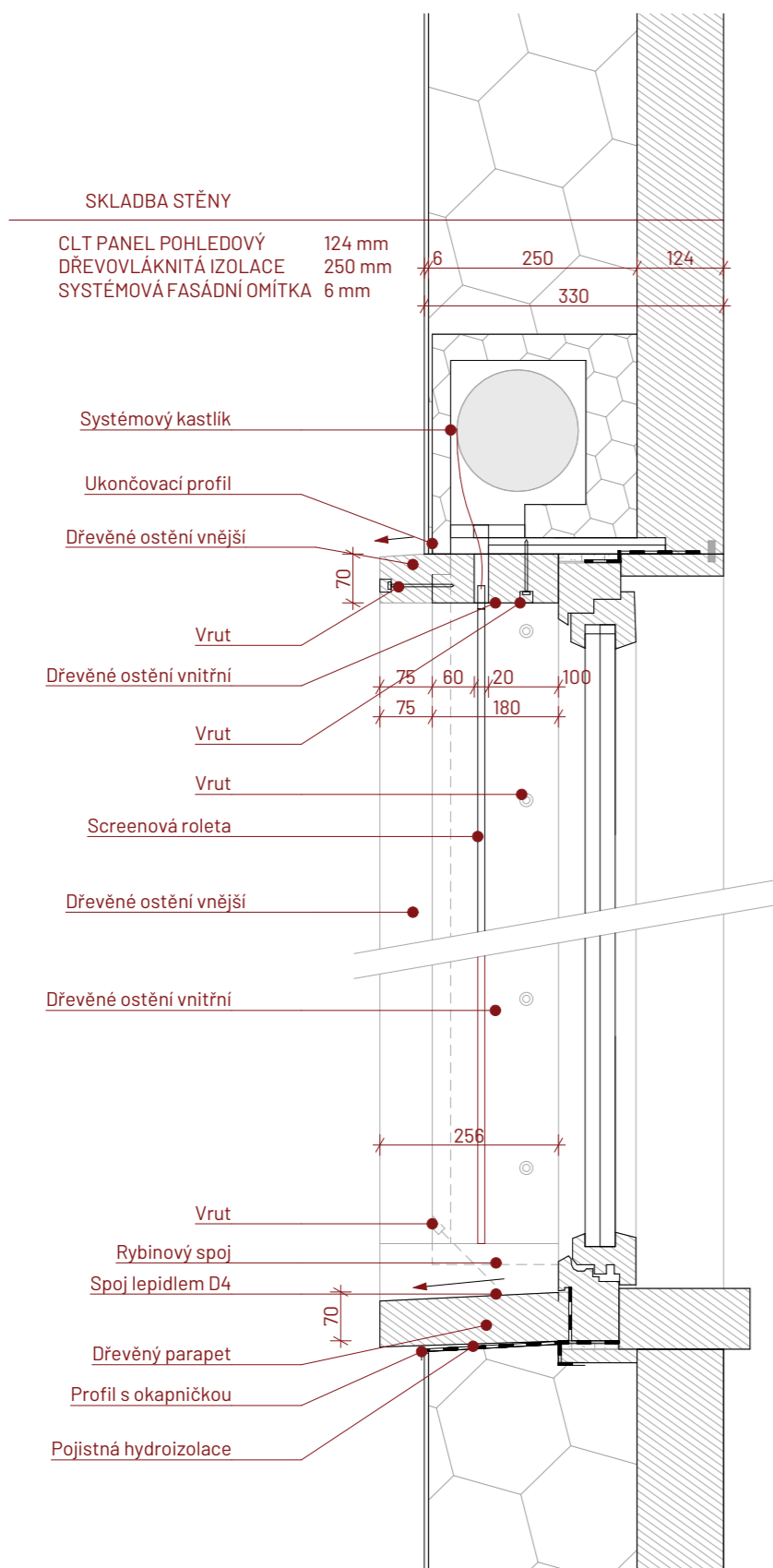
DETAIL OSTĚNÍ_M1:10
