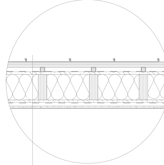
SKLADBA STRECHY
