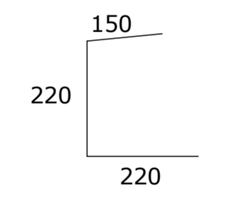
UZAVÍRACÍ PROFIL
