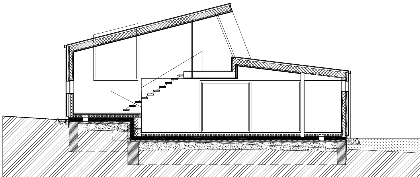
ŘEZ B-B
