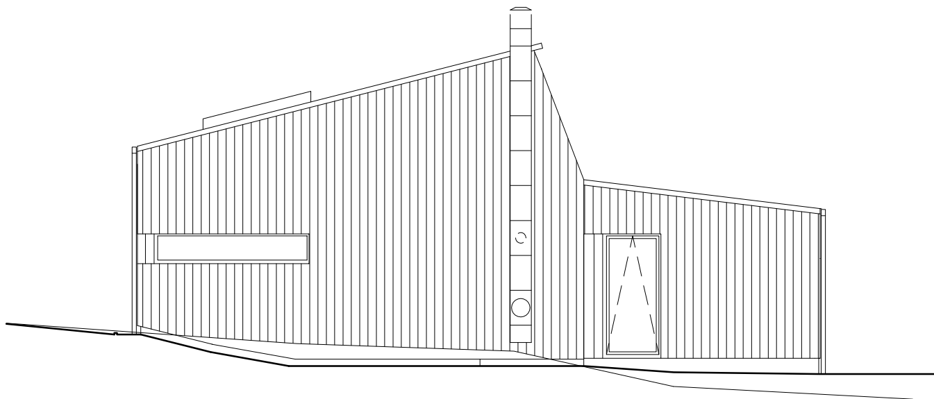
POHLED VÝCHODNÍ
