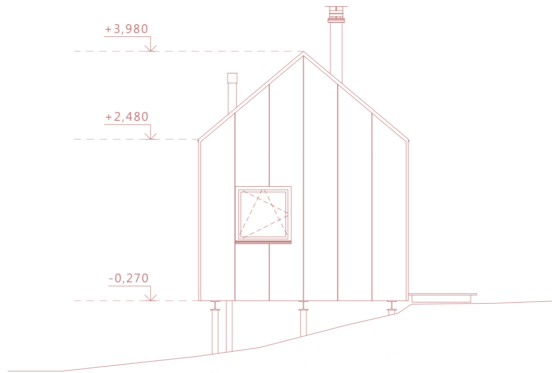
pohled - jižní
