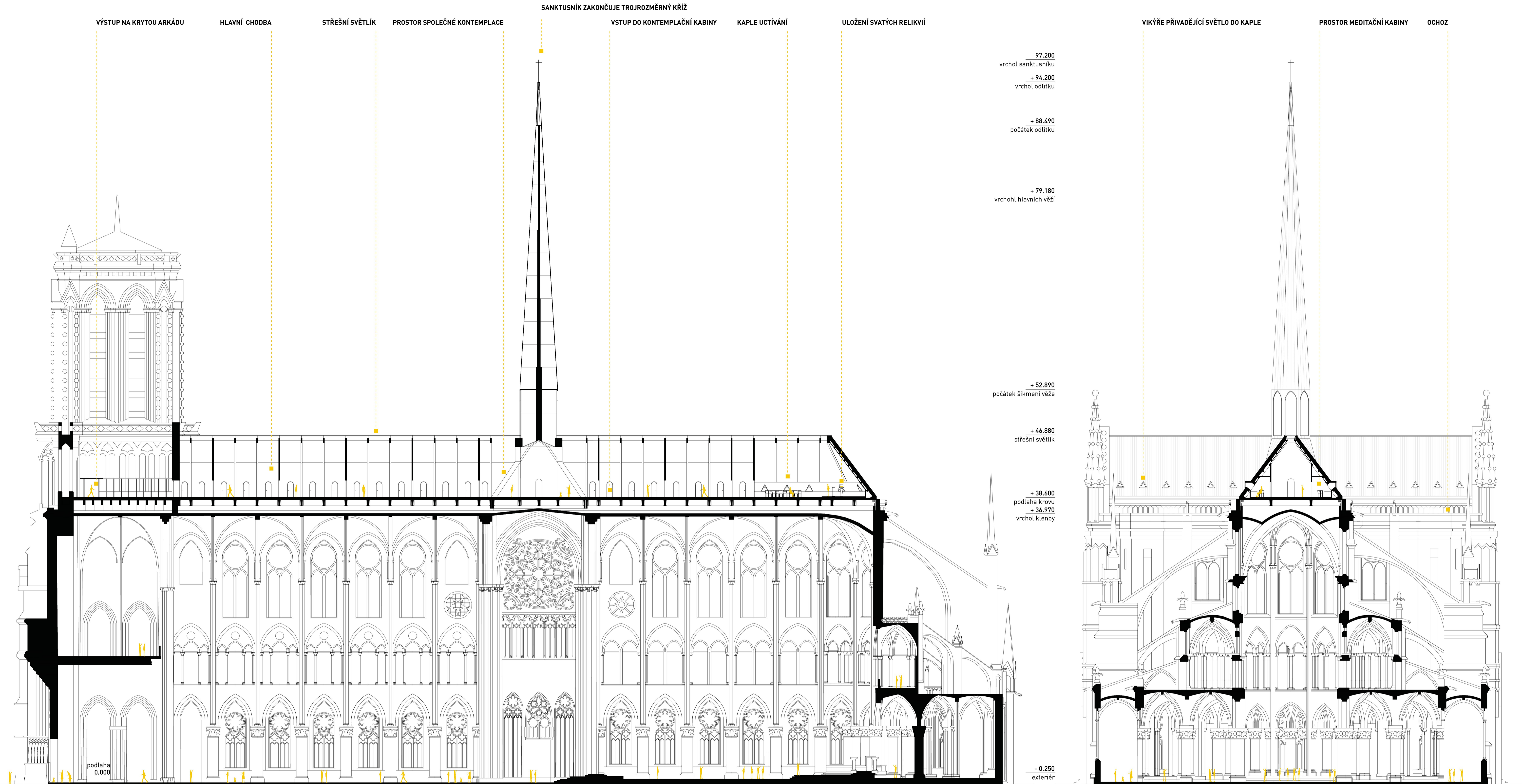
ŘEZ A - A
